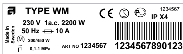
Muster Typenschild
